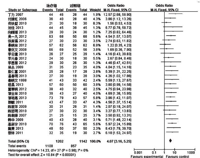
图1 两组患者有效率的Meta分析森林图
